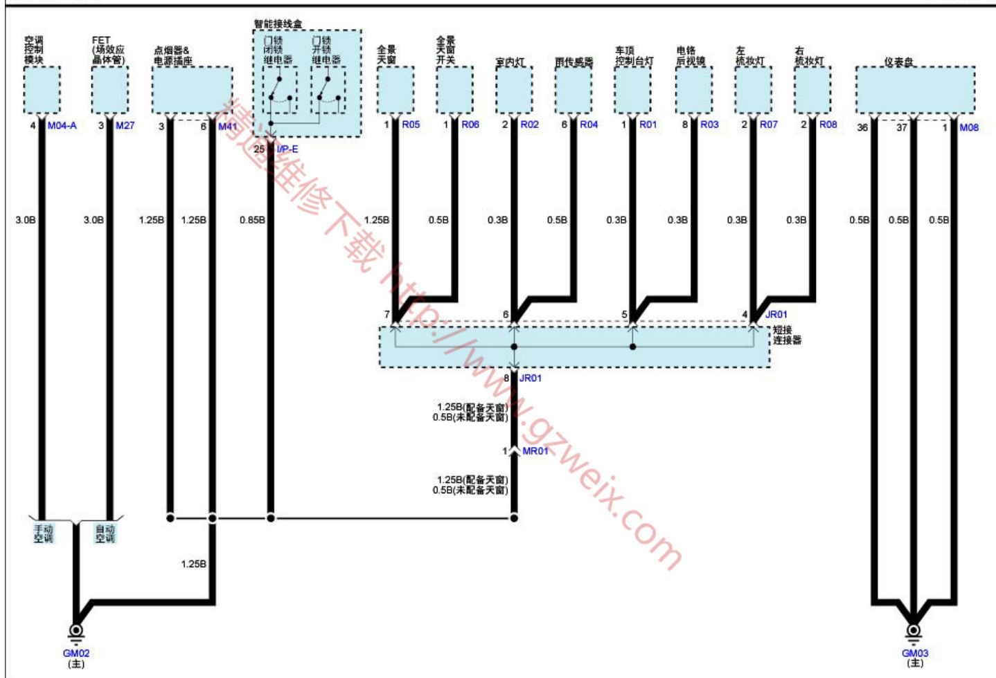
搭铁分布(2)
